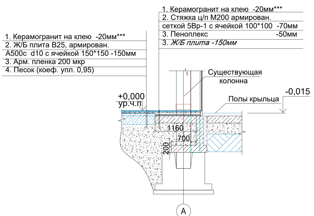
Схема устройства полов 1 этажа вдоль оси А
