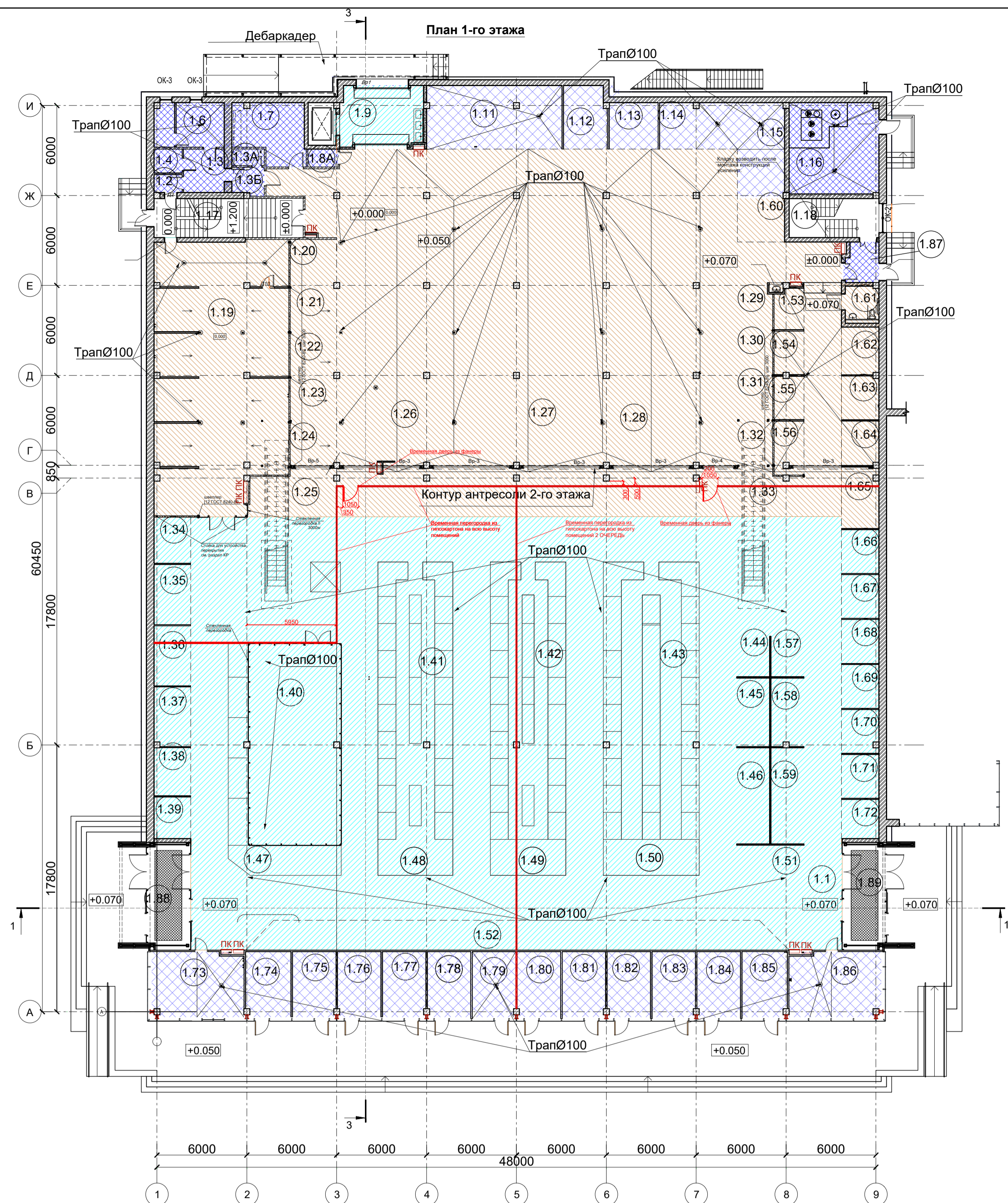
ЭКСПЛИКАЦИЯ ПОЛОВ на отм. +0.000 (1 этаж)
