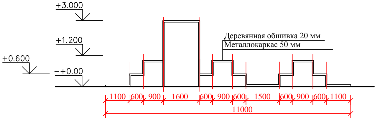
Вид А
