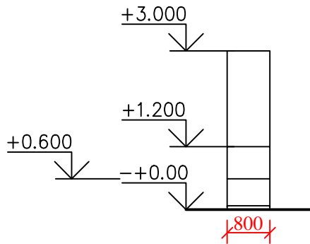
Вид Б
