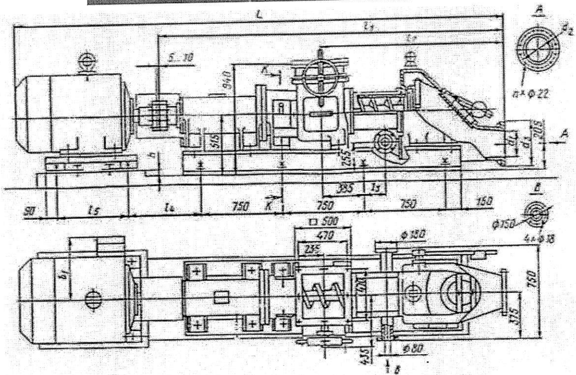
Рис. 1 Монтажно-габаритный чертёж
