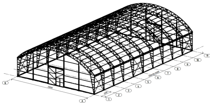
СХЕМА АНГАРА тип В
