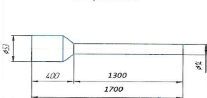
Эскиз электрозапальника
