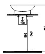
GÖVDE ÜSTÜ LAVABO BATARYA DELİKLİ TAŞMA DELİKLİ HRLG04601FD1W5000 460x550 mm
