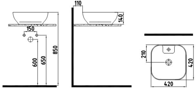
MOTTO KARE GÖVDE ÜSTÜ LAVABO BATARYA DELİKLİ/TAŞMA DELİKSİZ MTLG04201FD1W5000 420x420 mm Beyaz 679 TL
