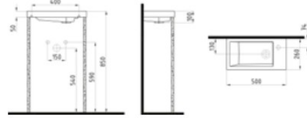
DOLAP UYUMLU LAVABO INLK05001FD1W5000 500x260 mm Taşıma deliksiz.
