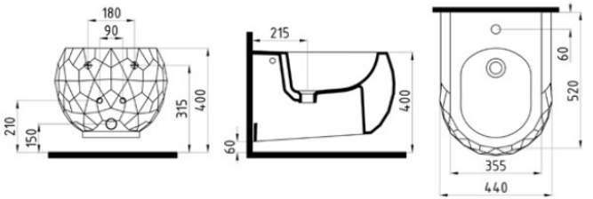
ASMA BİDE PNBA05201VD1W3000 520x350 mm
