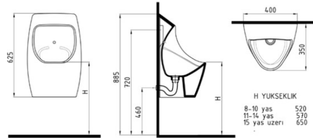
HARMONY PİSUAR 62 CM ARKADAN SU GİRİŞLİ ANK. FOTOSELLİ YIKAMA HRPS06203VSAW5000
