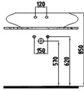
GÖVDE ÜSTÜ LAVABO BATARYA DELİKLİ TAŞMA DELİKLİ HRLG08001FD1W5000 800x510 mm
