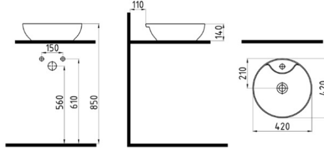
GÖVDE ÜSTÜ LAVABO BATARYA DELİKLİ / TAŞMA DELİKSİZ MTLG04202FD1W5000 Ø 420 mm
