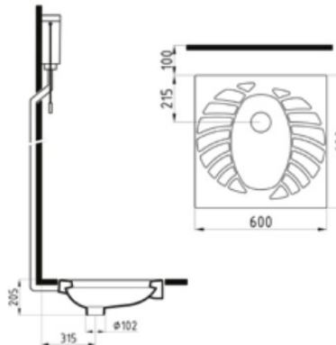
ÇEVRE YIKAMALI AY HELA TAŞI TPHT06001VSAW5000 600x600 mm Arkadan su girişli.
