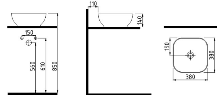
GÖVDE ÜSTÜ LAVABO BATARYA DELİKSİZ / TAŞMA DELİKSİZ MTLG03801FD0W5000 380X380 mm
