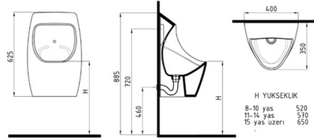
HARMONY PİSUAR 62 CM ARKADAN SU GİRİŞLİ+NOZZLE ANK. FOTOSELLİ YIKAMA HRPS06203VSAW5000
