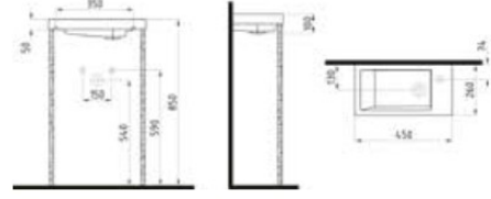
DOLAP UYUMLU LAVABO INLK04501FD1W5000 450x260 mm Taşıma deliksiz.
