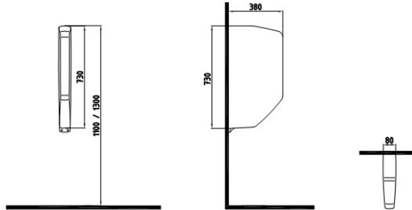
PİSUAR ARA BÖLME NPPA07301V00W5000 730x380 mm Beyaz 489 TL
