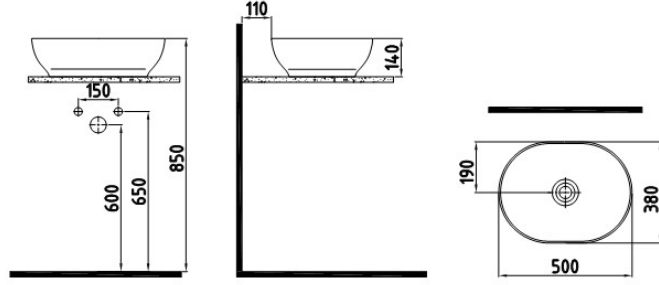
GÖVDE ÜSTÜ LAVABO BATARYA DELİKSİZ / TAŞMA DELİKSİZ MTLG05001FD0W5000 500x380 mm
