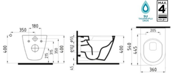
ASMA KLOZET NO-RİM ALKA054H1VP1W5000 540x360 mm
