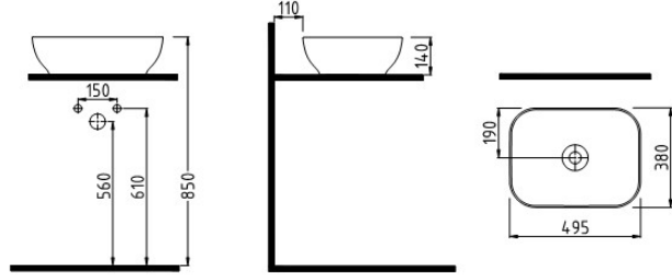
GÖVDE ÜSTÜ LAVABO BATARYA DELİKSİZ TAŞMA DELİKSİZ MTLG05003FDOW5000 495x380 mm
