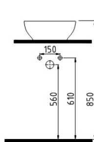
GÖVDE ÜSTÜ LAVABO BATARYA DELİKSİZ / TAŞMA DELİKSİZ MTLG03802FD0W5000 Ø 380 mm
