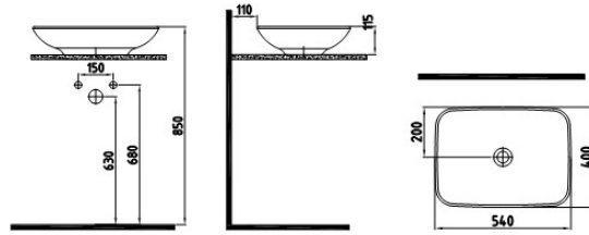
GÖVDE ÜSTÜ DİKDÖRTGEN LAVABO BATARYA DELİKSİZ TAŞMA DELİKSİZ HRLG05401FDOW5000 540x400 mm
