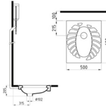
ÇEVRE YIKAMALI AY HELA TAŞI TPHT05001VSAW5000 500x600 mm Arkadan su girişli.
