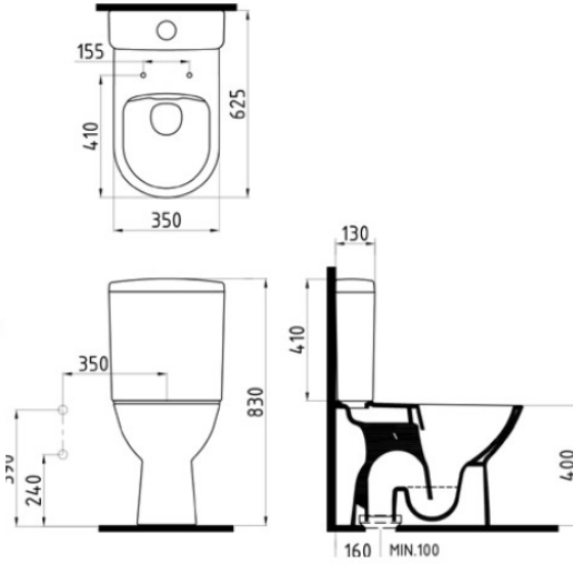
REZERVUAR CPRS04101VDAW5000 (Orion-Venüs klozetlerle uyumludur) 410x370 mm
