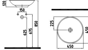
GÖVDE ÜSTÜ ÇANAK LAVABO BATARYA DELİKSİZ TAŞMA DELİKSİZ HRLG04501FDOW5000 Ø450
