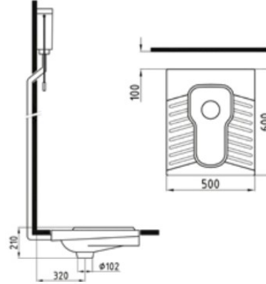
ÇEVRE YIKAMALI HELA TAŞI TPHT05002VSAW5000 500x600 mm Arkadan su girişli.
