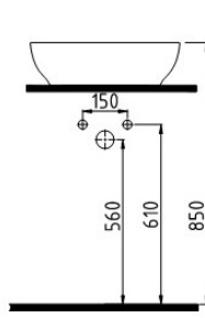
OVAL GÖVDE ÜSTÜ LAVABO BATARYA DELİKSİZ / TAŞMA DELİKSİZ MTLG05002FD0W5000 495x375 mm
